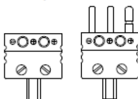
Gniazdo i wtyk STANDARD linia 3-przewodowa
