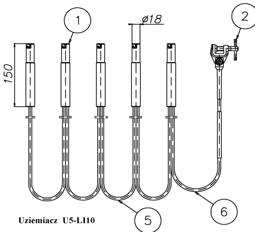
Uziemiacz U5-LI10
