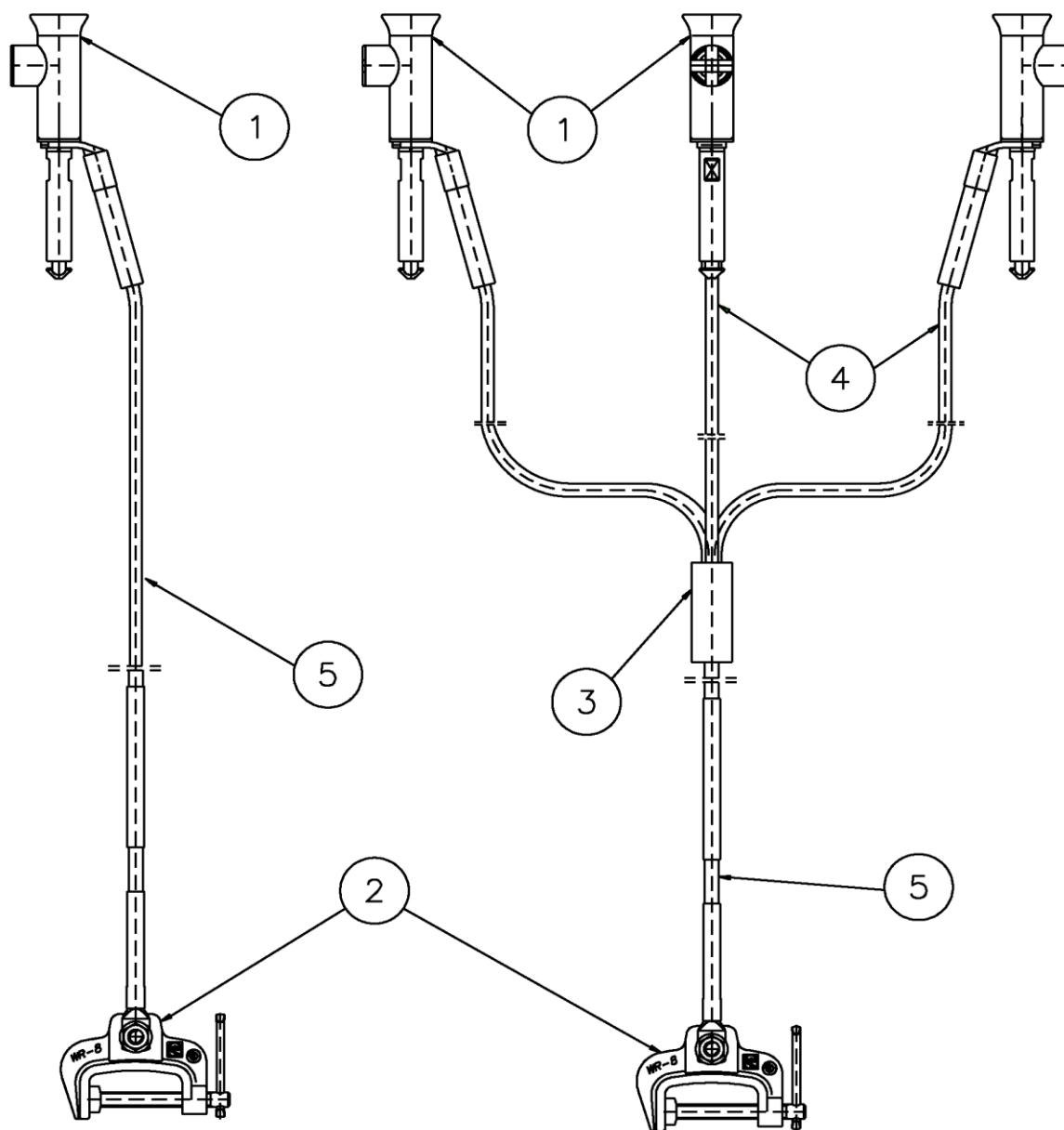
Uziemiacz U1-S
